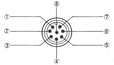
コネクター接続図[外側から見た図]
