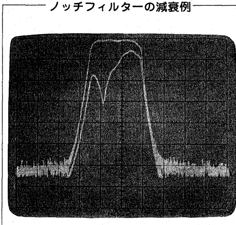
ノッチフィルターの減衰例
